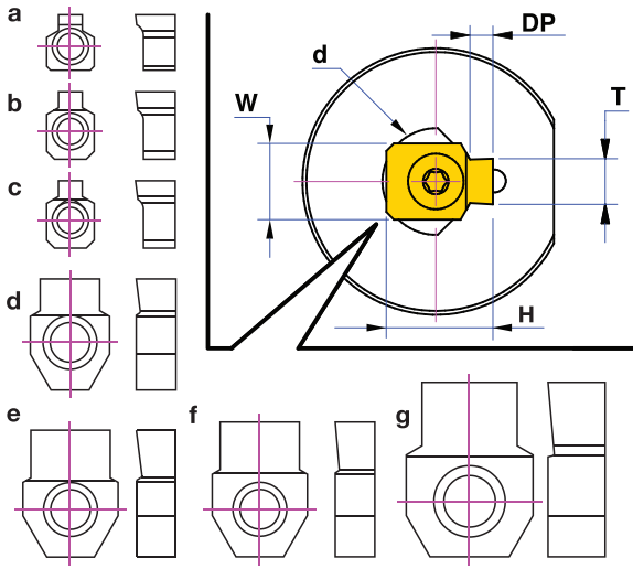
Insert dimensions
